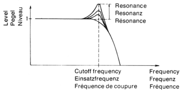
VCF-Frequenzempfindlichkeit
